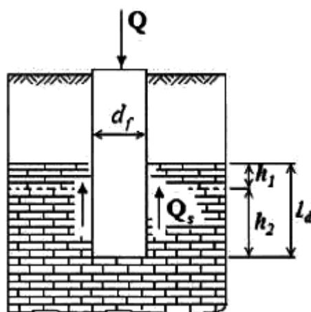
Рисунок Б.1 - Прорезание свай толщ скальных грунтов
