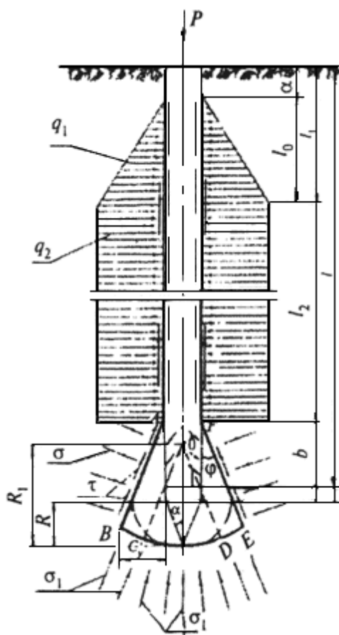
Рисунок Е.1 - Расчетная схема
