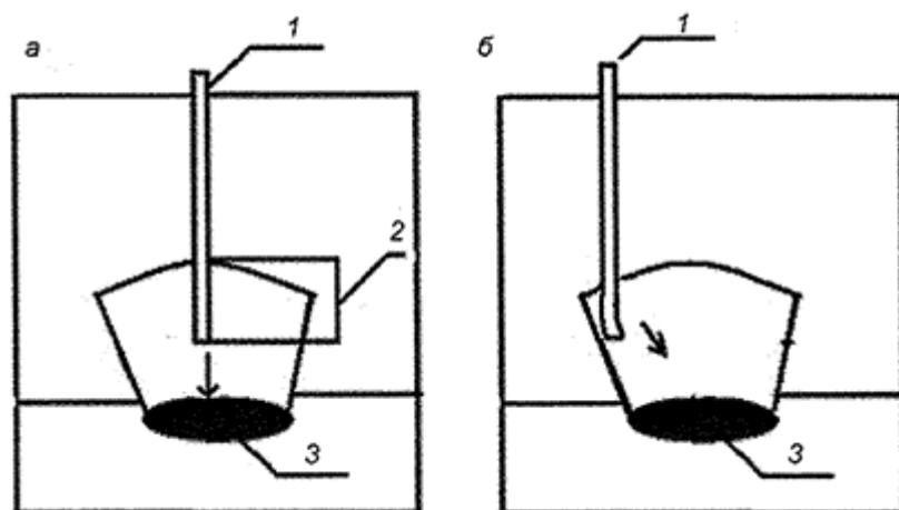
Рисунок 3 - Схемы механического взаимодействия свай с карстовыми полостями
