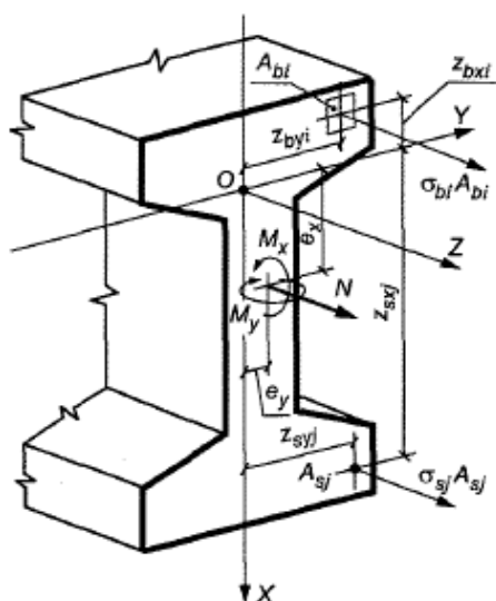
Рисунок 8.5 - Расчетная схема нормального сечения железобетонного элемента
